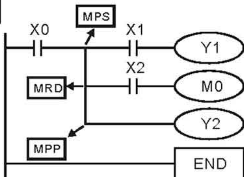
Релейно-контактная схема
