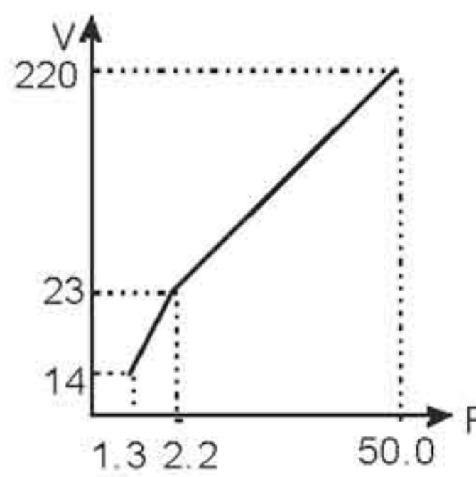
Двигатель 60Гц
