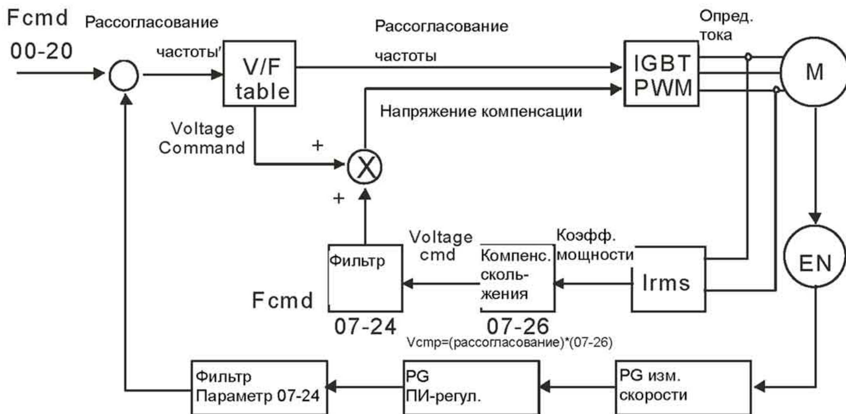
Блок-схема режима V/f управление + Энкодер (параметр 00-11 = 1).
