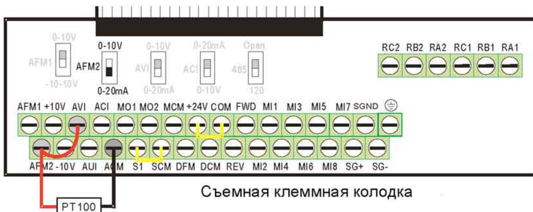
Схема подключения PT100:
