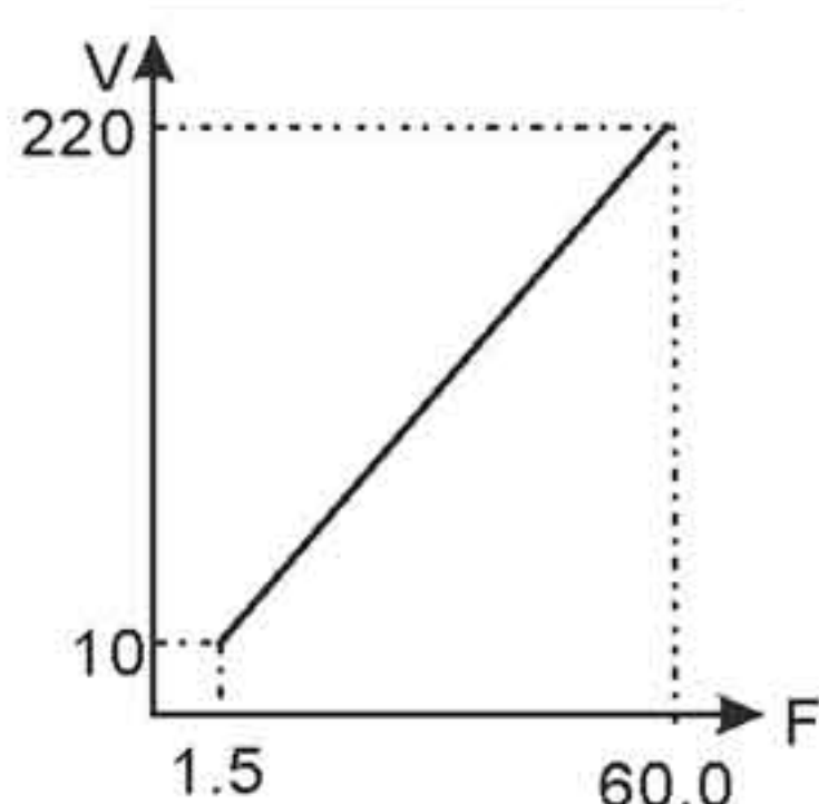
Двигатель 60Гц
