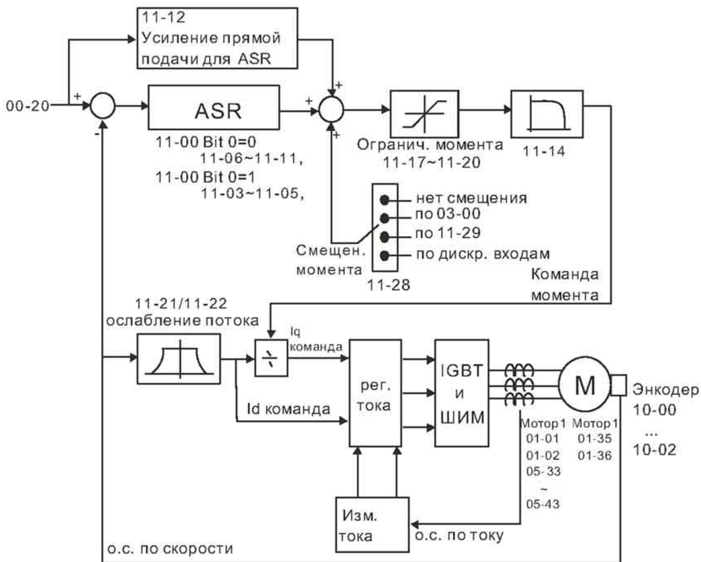
Блок-схема режима FOCPG для двигателя с постоянными магнитами (параметр 00-11 = 4).
