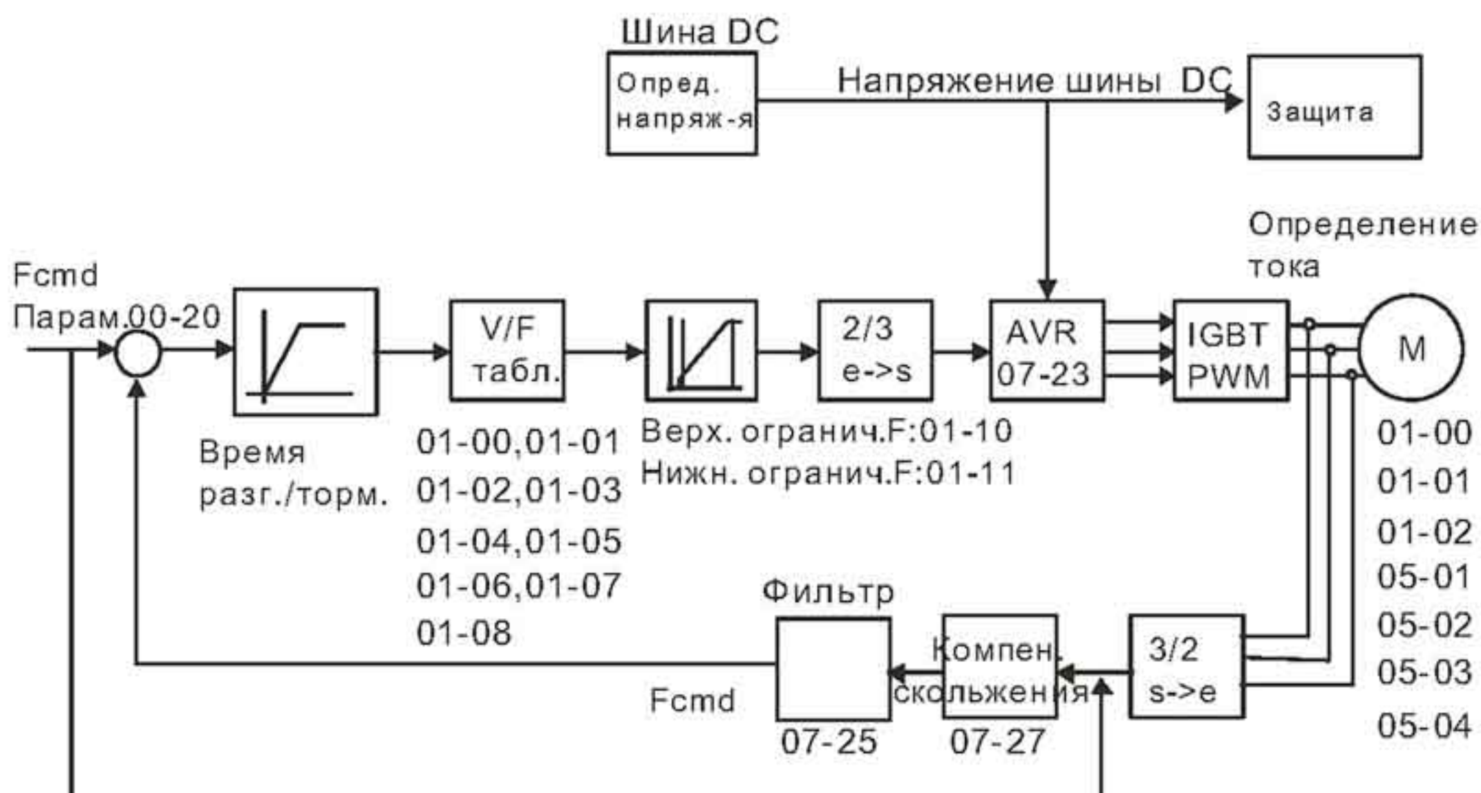
Блок-схема режима векторного управления без датчика (параметр 00-11 = 2).
