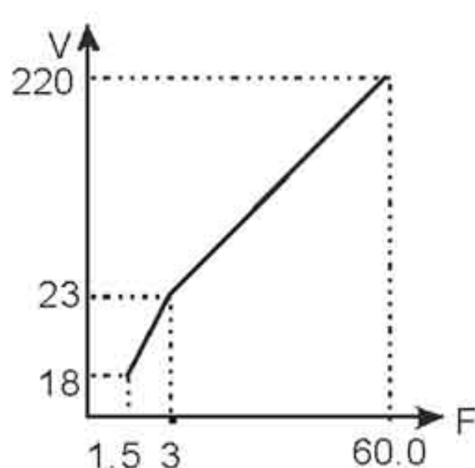
Двигатель 60Гц
