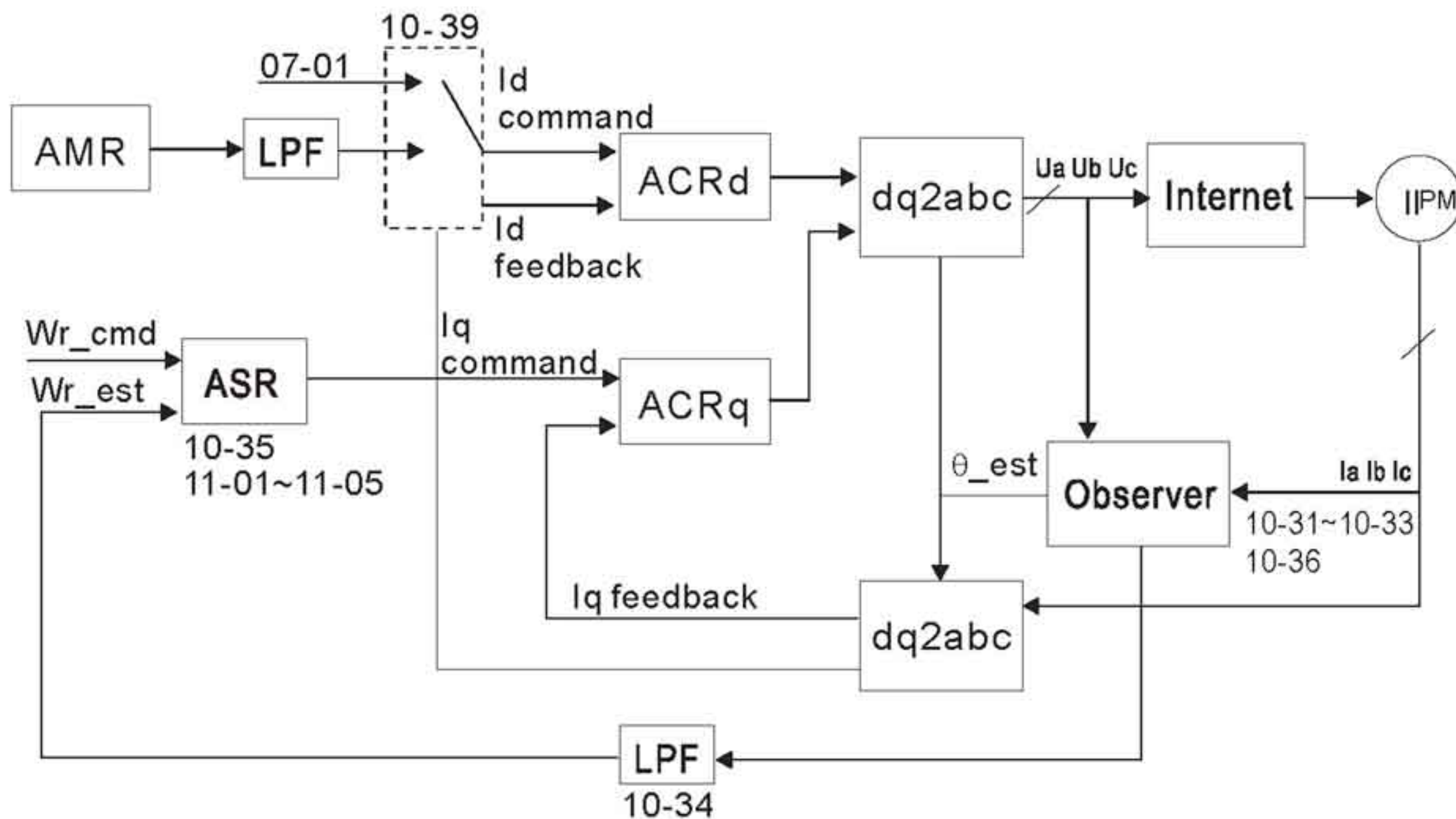
Блок-схема режима PM FOC (расширенное векторное управление двигателем с постоянными магнитами без датчика) (параметр 00-11 = 6).
