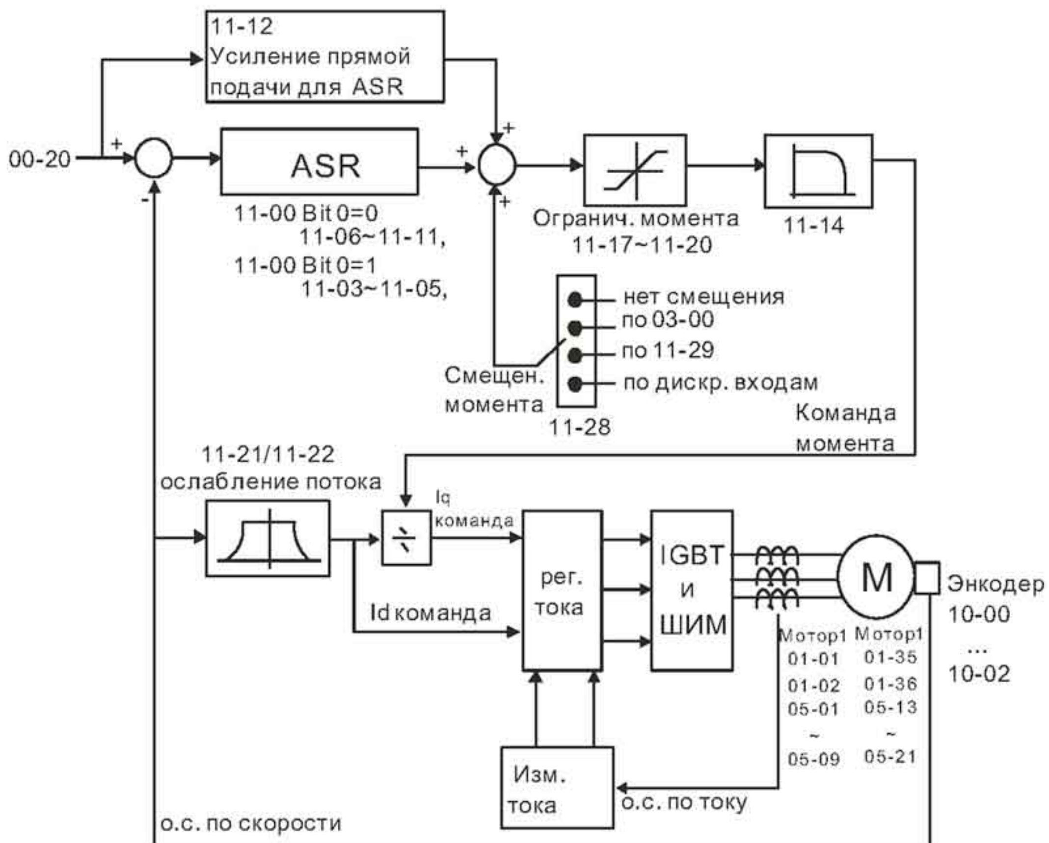
Блок-схема режима FOCPG (параметр 00-11 = 3).
