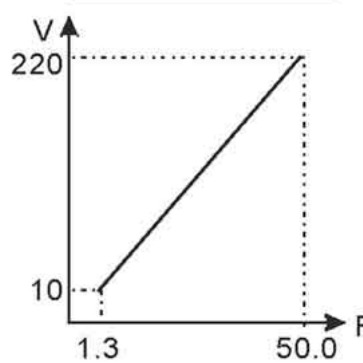
Двигатель 50 Гц
