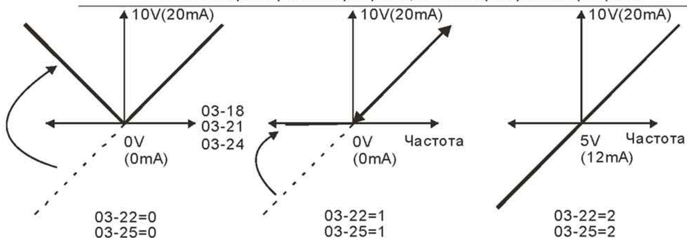
Аналоговый выходной сигнал при реверсе
