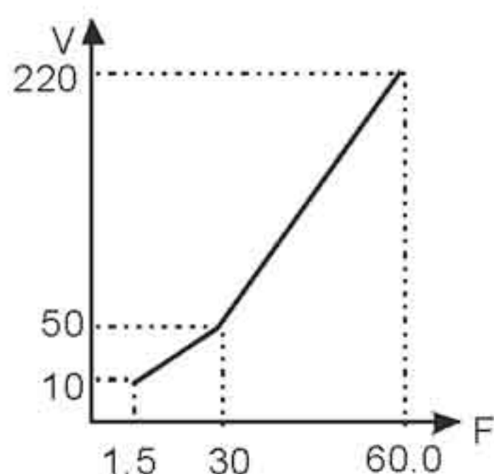
Двигатель 60Гц
