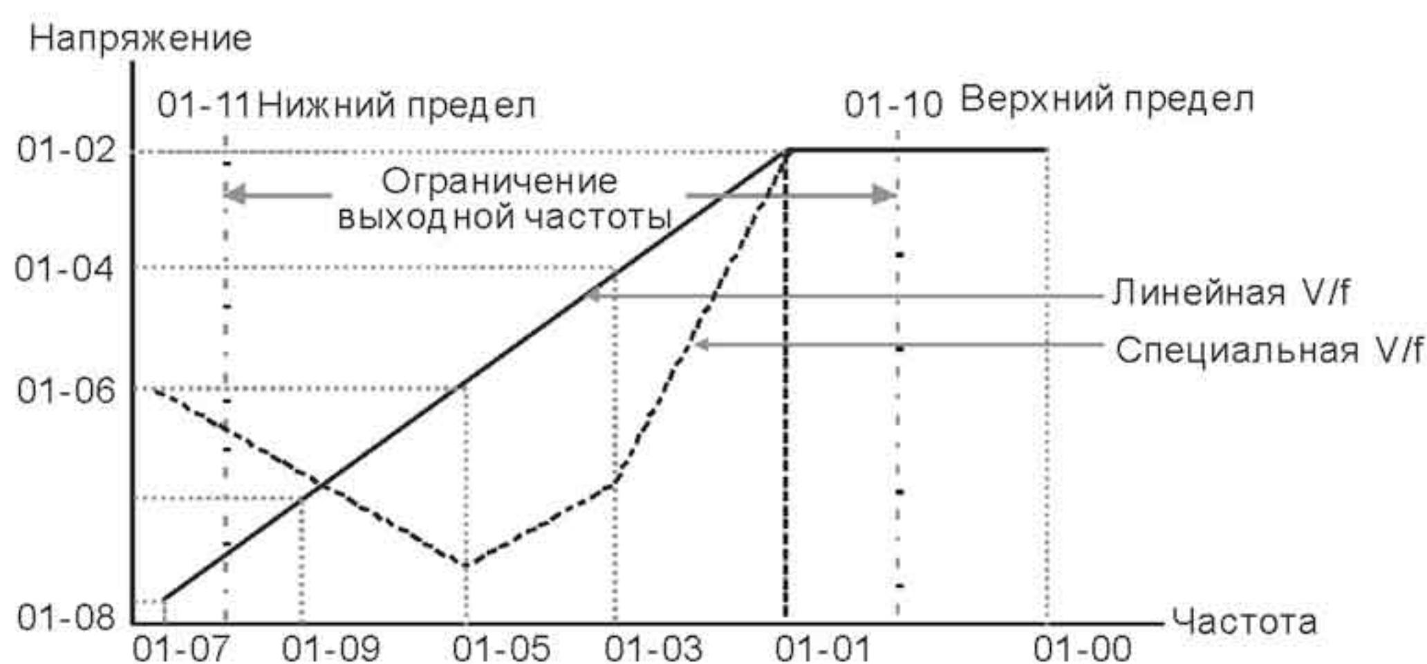
Вольт-частотная (V/f) характеристика привода
