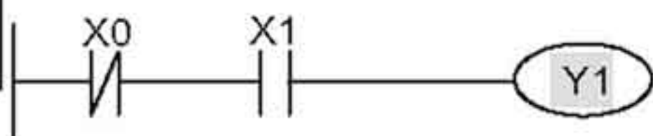
Релейно-контактная схема
