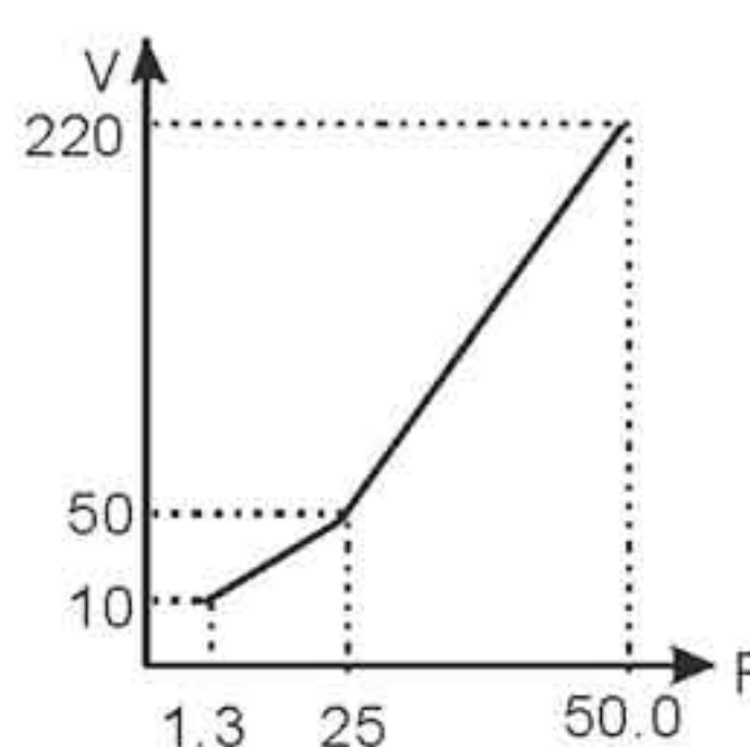
Двигатель 50Гц
